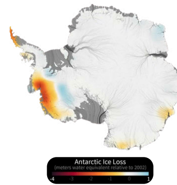
Carte de la fonte de la glace en Antarctique en seulement 20 ans
